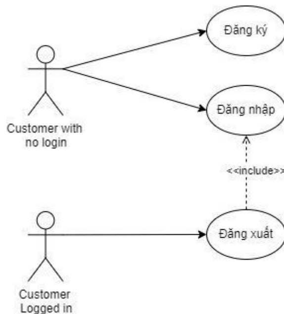
Hình 3. 1 Use-case đăng nhập, đăng ký, đăng xuất
